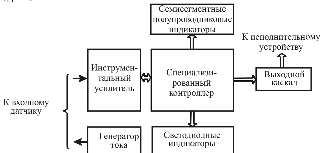
Рисунок 2 - Функциональная схема прибора
